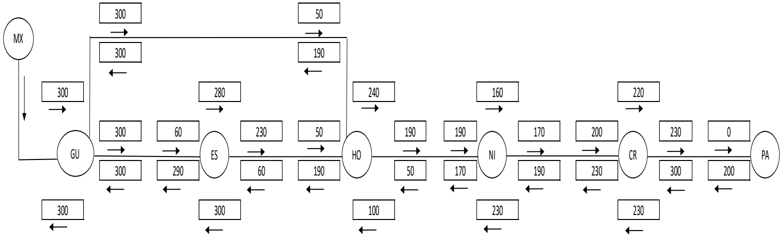
Diagrama 11.1- Valores individuales de MCTP (Porteo, Importación y Exportación) más restrictivas para DT
