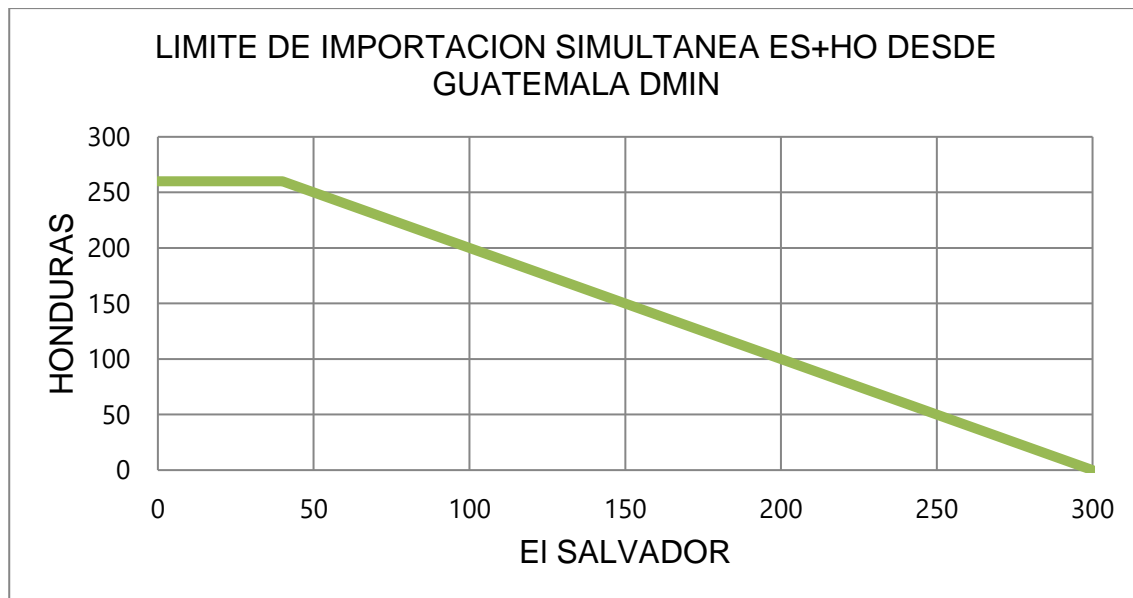
Gráfica 3. Restricción importación simultánea de El Salvador y Honduras– demanda mínima
